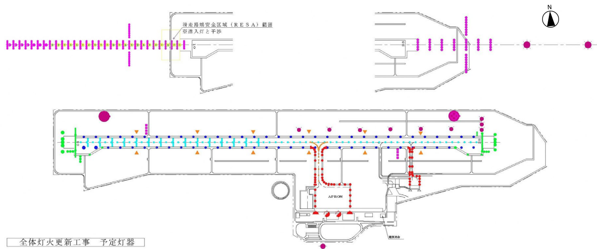
航空灯火の更新計画(約700基余り) 配置図
